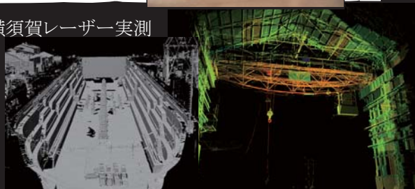
旧横須賀海軍工廠建物の実測調査
