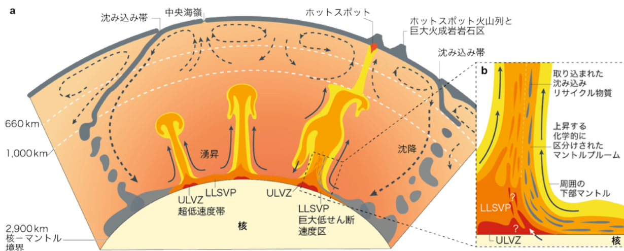
図1. 地球の内部構造(Koppers et al., 2021 の Fig. 1 を日本語訳)
