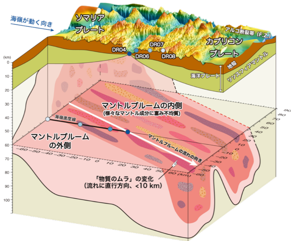
図4. レユニオンマントルプルームによってもたらされた上部マントルの不均質構造
