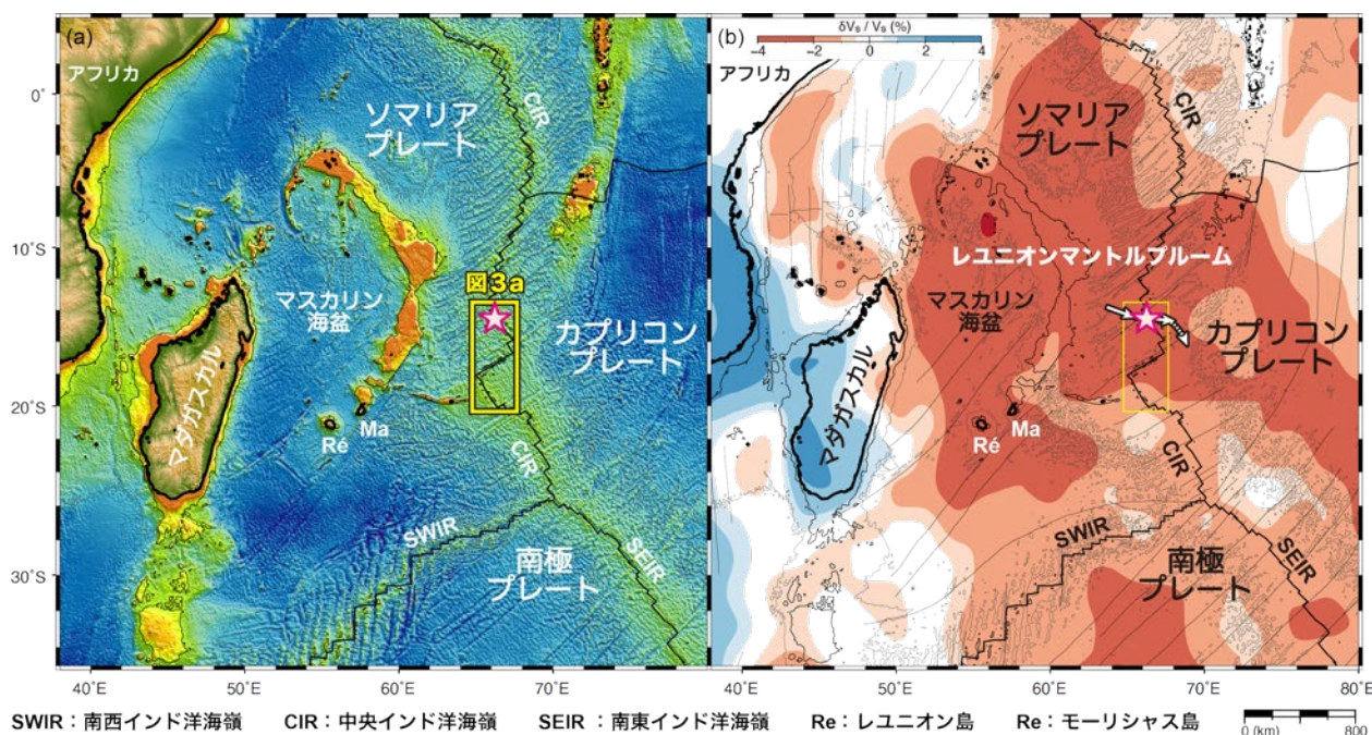
図2. 中央インド洋海嶺とレユニオンホットスポットにおける「海嶺－ホットスポット相互作用」
