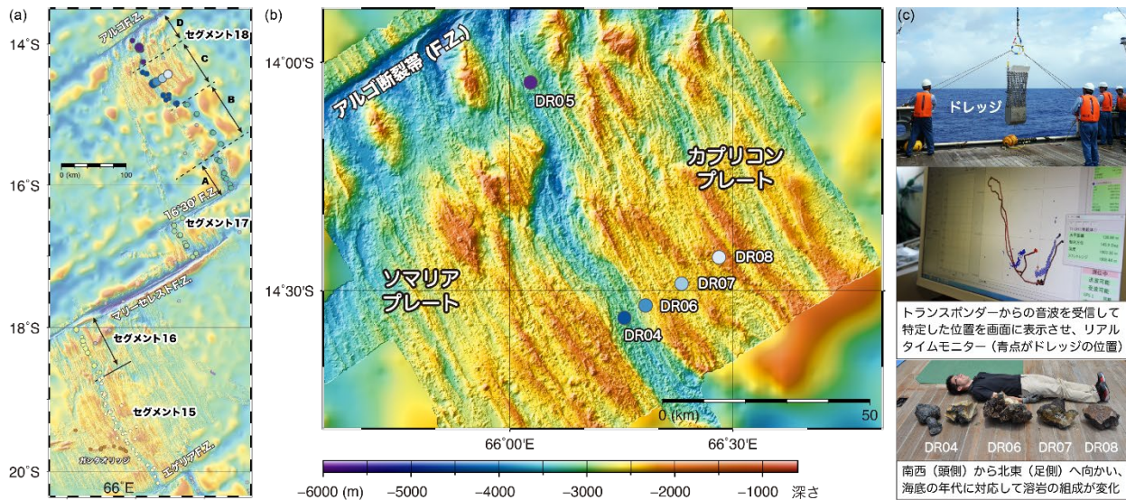
図3. 本研究対象海域のサンプル採取地点とドレッジ
