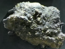
黄銅鉱
