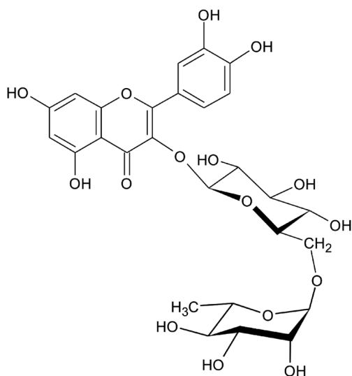
Fig. 3. Quercetin 3- O -rutinoside ( 2 , rutin).
