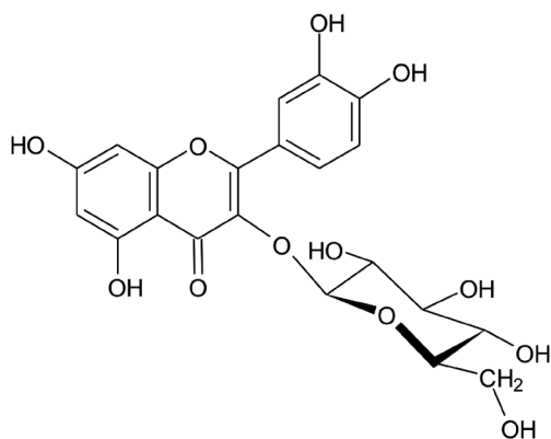
Fig. 4. Quercetin 3- O -glucoside ( 3 , isoquercitrin).
