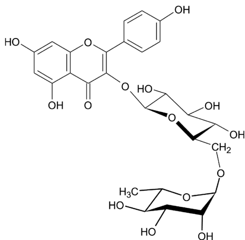
Fig. 5. Kaempferol 3- O -rutinoside ( 4 , nicotiflorin).
