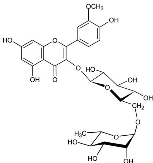
Fig. 6. Isorhamnetin 3- O -rutinoside ( 5 , narcissin).
