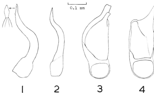
Figs. 1–4. Aedeagi of Corticariinae. — 1, Melanophthalma ( Cortilena ) sakagutii sp. n., lateral, with ventral view of apex; 2, M. (s. str.) japonica sp. n., lateral; 3, Corticarina khnzoriani sp. n., ventral; 4, C. nakanei sp. n., ventral.
