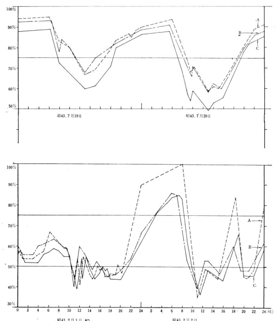
図5. 湿度の日変化の比較 A: 苗畑 B: 実験畑 C: 食草園
