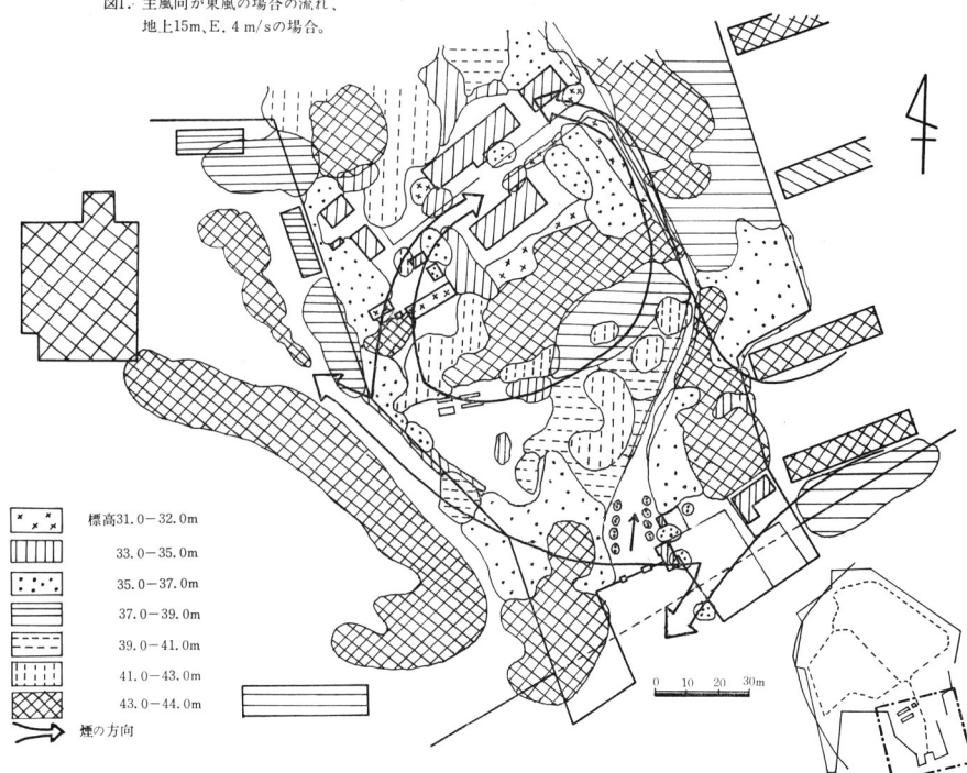
図2. 主風向が北風の場合の流れ、 地上15m, N.NE, 6 m/sの場合。
