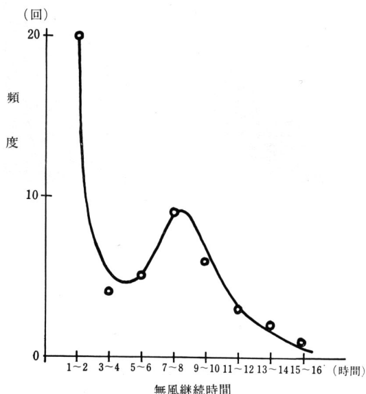
第29図 無風継続状況(1970.10.30～6.12)
