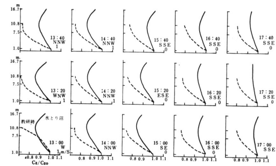
第21図 自然教育園のCO 2 垂直分布(1970.11.5)
