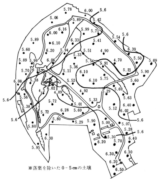
第23図 自然教育園PH分布図(1971.12.4-12)
