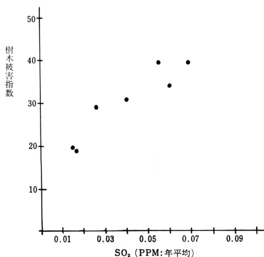
第1図 樹木被害とSO 2 の関係
