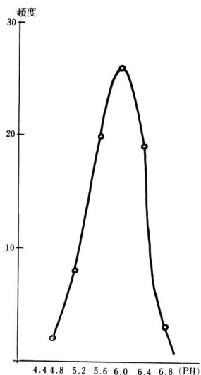
第24図 自然教育園における PHの分布 (1971. 12. 4—12 (0—5.0cm))
