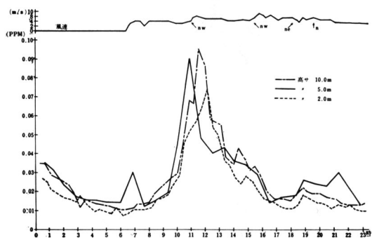
第18図 SO 2 の日変化（1971. 7月15日快晴） 於教研跡
