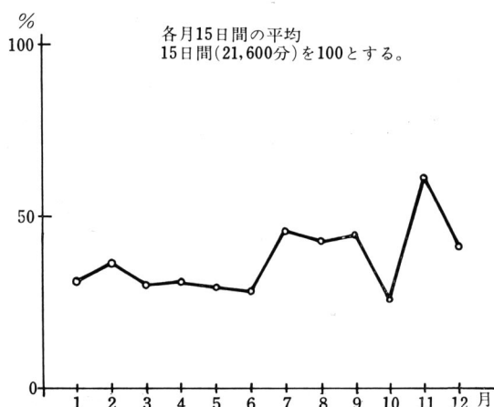
第28図 各月の無風時間(1969年' 於水とり沼)
