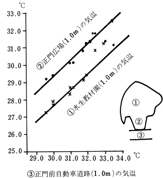
第27—3図 自然教育園内外の気温差
