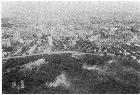
写真4 発煙による気流調査
