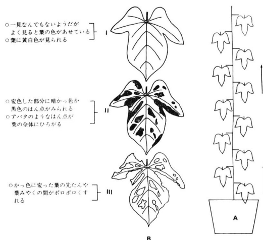
図3 被害度区分と記録方法
