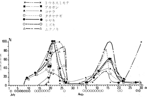
図16 異常落葉日変化
