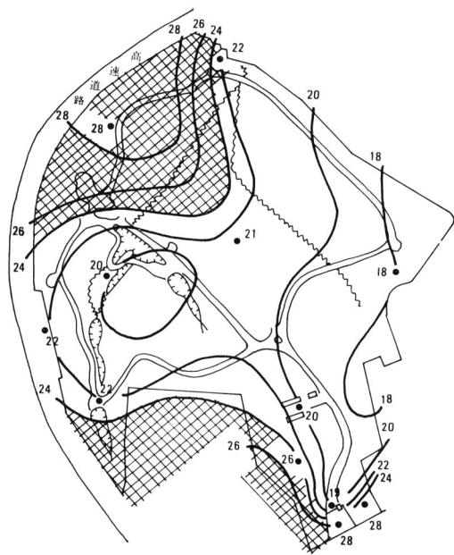
図9 アサガオ葉被害分布(第2回) 1973, 7/28~8/3
