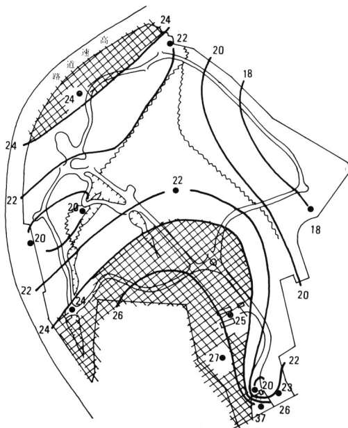
図8 アサガオ葉被害分布(第1回) 1973, 7/15~20
