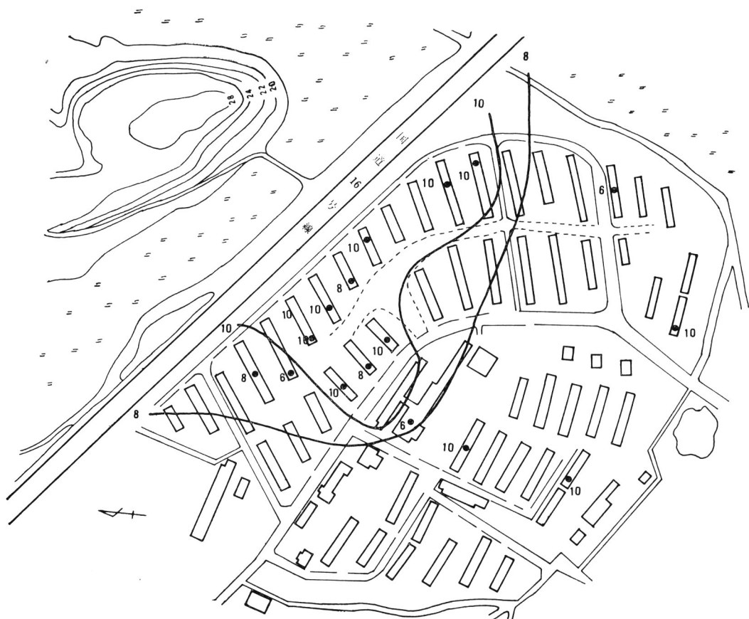
図14 千草台団地、アサガオ葉被害分布図(大賀.1973.未発表)
