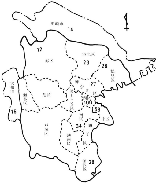
図12 横浜市内，アサガオ葉被害分布図（1973. 8. 31） ※資料提供，神奈川県科学センター ※数値は総葉数に対する被害葉率（％）
