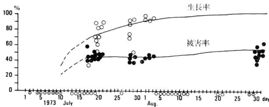
図5 生長率曲線と被害率
