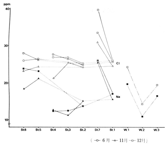
図 3 Cl, Na の変動
