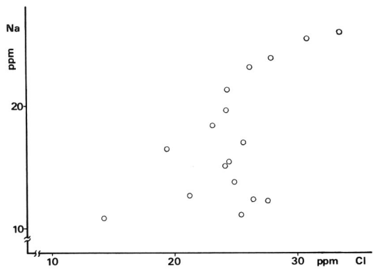
図 6 Na と Cl 含量の相関
