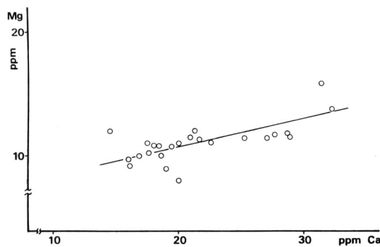
図 5 Mg と Ca 含量の相関
