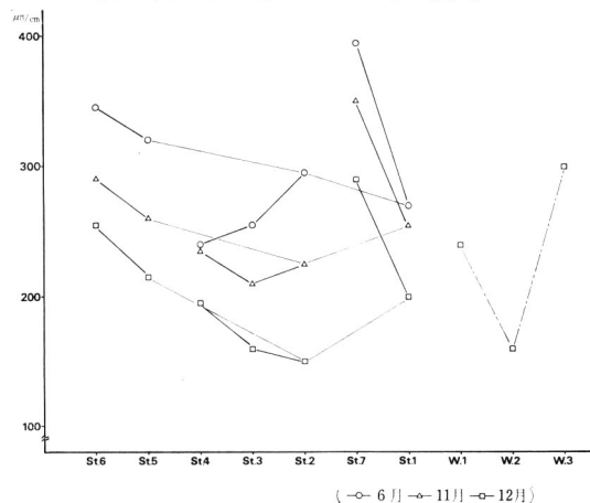
図12 電導度の変動
