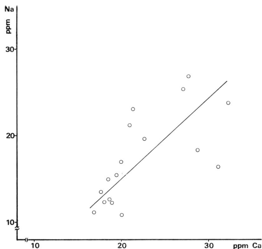
図7 NaとCa 含量の相関
