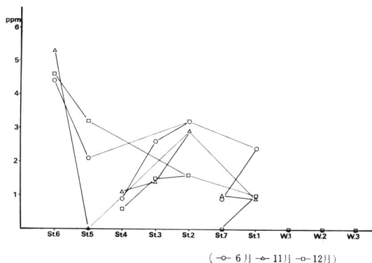
図9 BOD の変動
