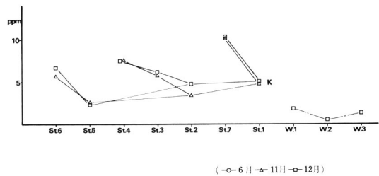
図 4 K の変動
