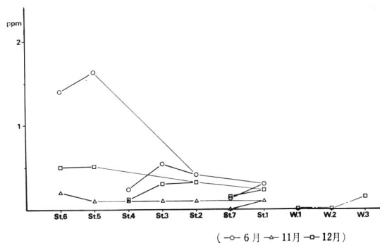
図8 \text{NH}_4^+\text{-N} の変動
