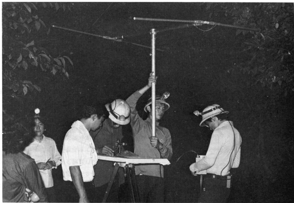
図2 発信器の着装と方探による調査のようす
