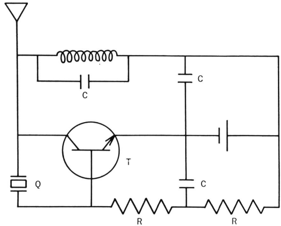
図3 発信機配線図
