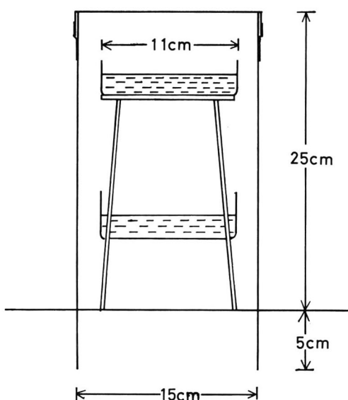
図 1 土壤呼吸速度測定装置の概略図
