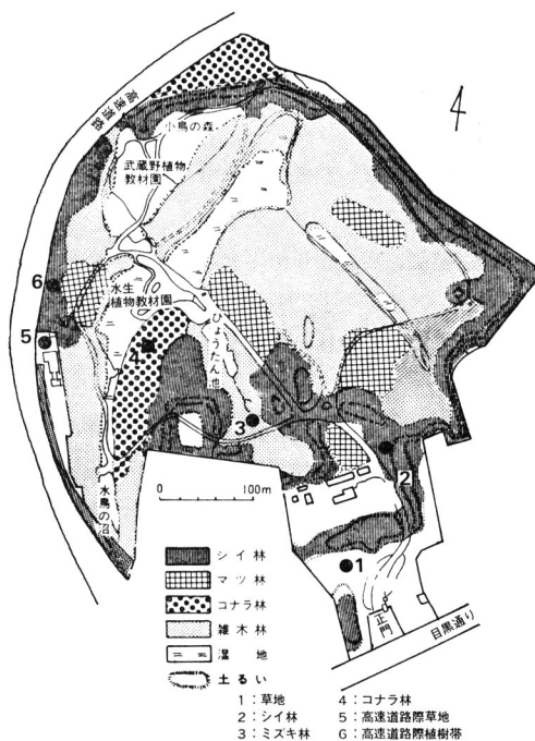
図3 降下媒塵の測定地点
