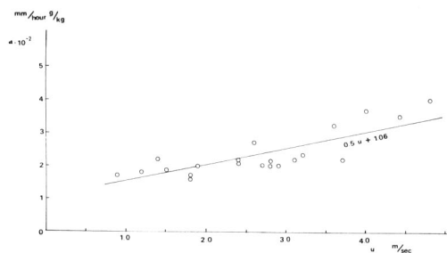
図6 蒸発傾度 ( \alpha ) と風速 ( u ) の関係
