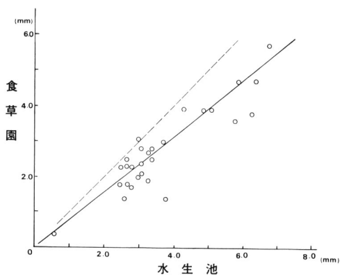
図5 食草園と水生池における蒸発量の比較
