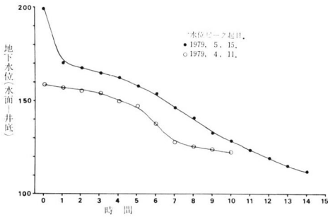
図 4. No. 7 観測孔の地下水位減少状況
