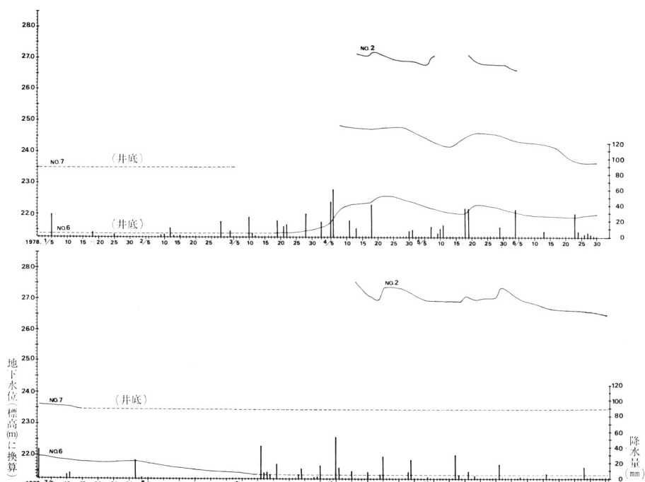
図 7. 地下水位変化状況 (1978)
