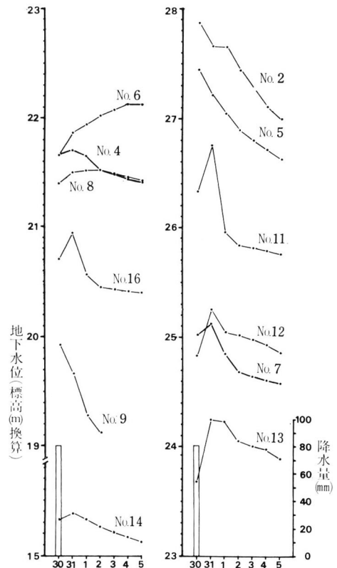
図 6. 降水量と地下水位変化
