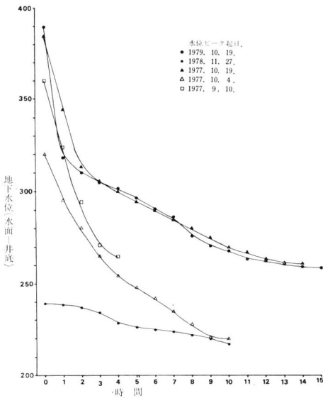
図 3. No. 2 観測孔の地下水位減少状況
