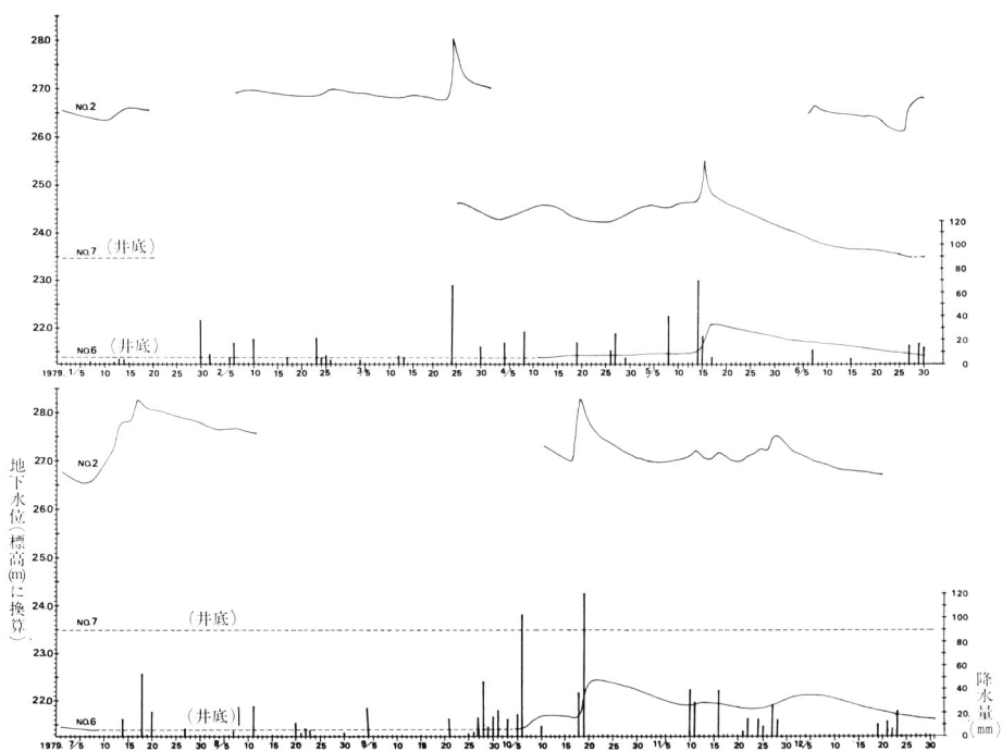
図 8. 地下水位変化状況 (1979)
