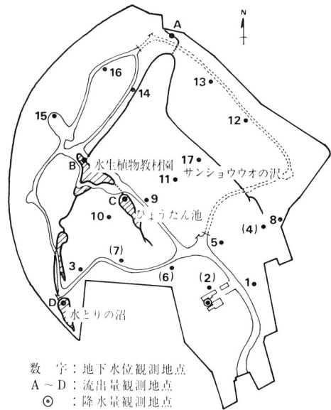
図 1. 地下水位、流量、降雨量の観測地点配置図
