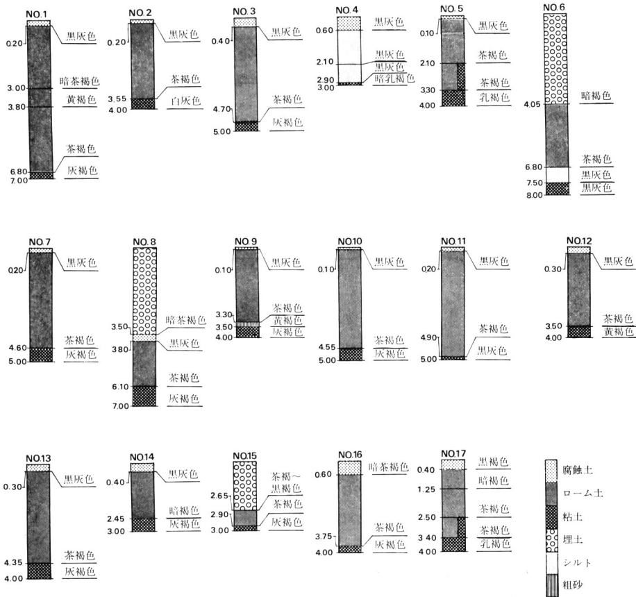
図 2. 地下水位観測孔の柱状図
