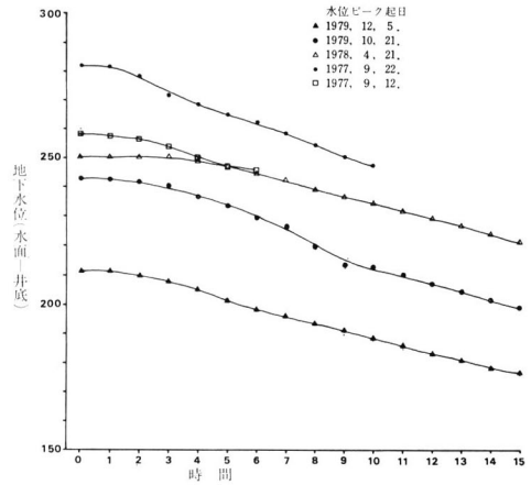
図 5. No. 6 観測孔の地下水位減少状況
