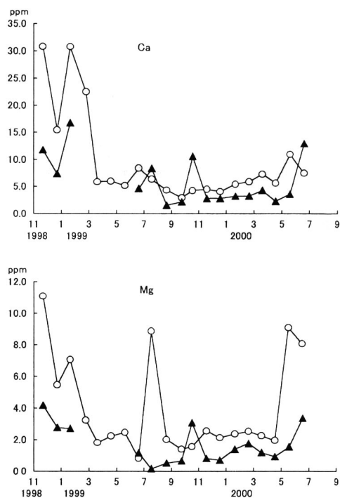
図7 林内雨のカルシウム, マグネシウム, カリウム濃度
