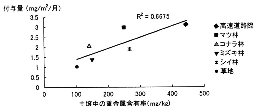
図11 Pbにおける降下ばいじんによる重金属の付与量と土壤中の重金属含有率の関係
