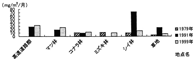
図7 Znの各地点の月当たり降下ばいじんによる重金属の付与量
