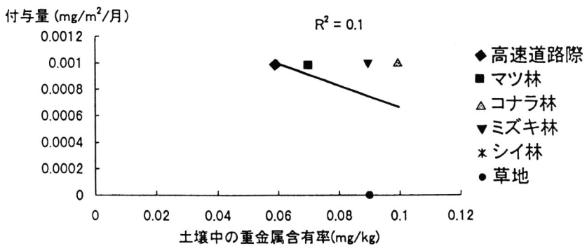
図10 Cdにおける降下ばいじんによる重金属の付与量と土壌中の重金属含有率の関係
