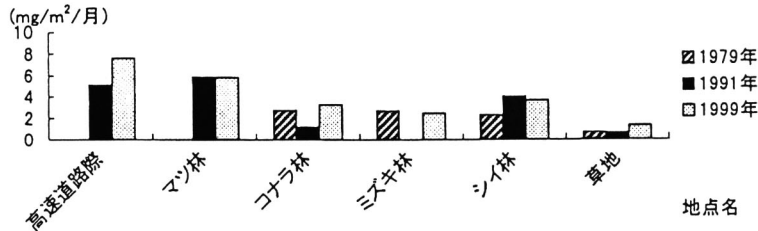
図5 Cuの各地点の月当たり降下ばいじんによる重金属の付与量
