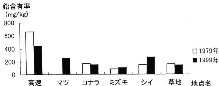
図3 1999年と1979年の鉛含有率比較
