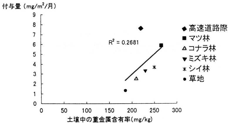
図9 Cuにおける降下ばいじんによる重金属の付与量と土壌中の重金属含有率の関係
