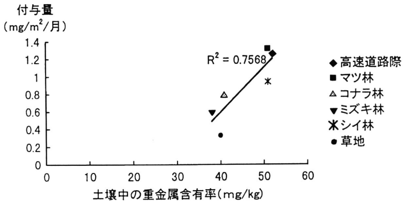
図8 Niにおける降下ばいじんによる重金属の付与量と土壌中の重金属含有率の関係
