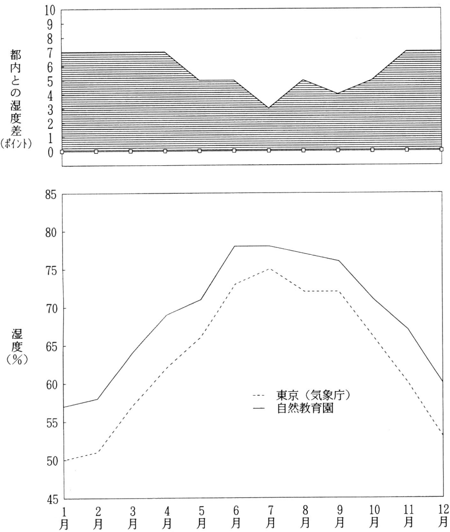
図 5. 自然教育園の平年湿度 (1971~2000年)
