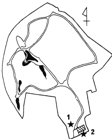
図1. 自然教育園の気象観測地点
