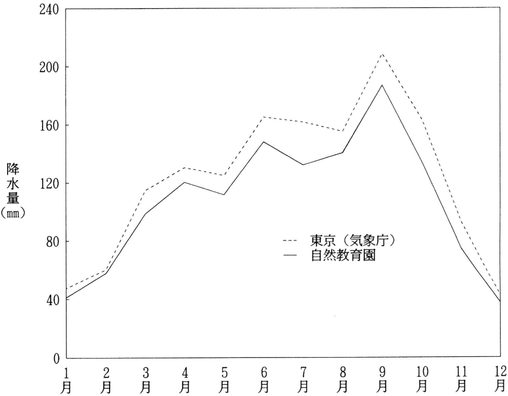
図 8. 自然教育園の平年降水量 (1971~2000年)
