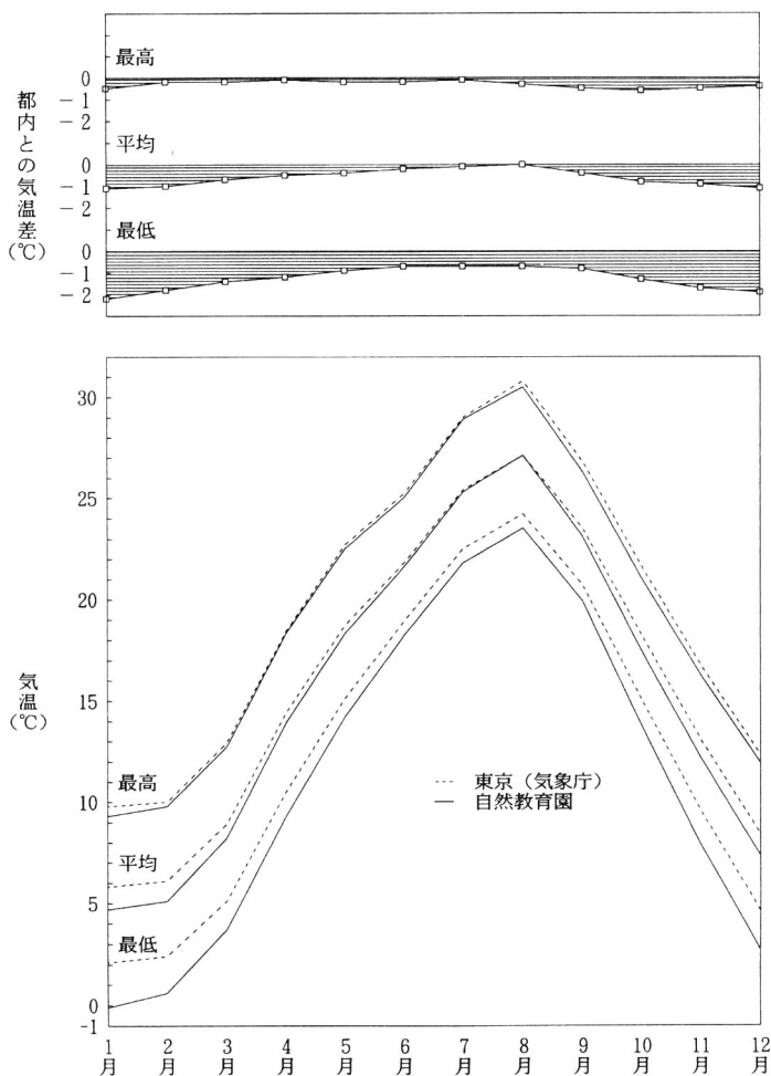
図 2. 自然教育園の平年気温 (1971~2000年)
