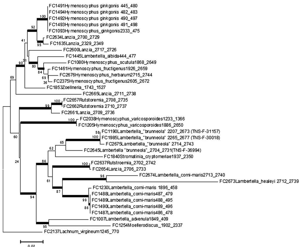
図3. Lambertella “ brunneola ” および Lambertella , Hymenoscyphus 属を中心とした ITS-5.8S およびリボソーム大サブユニット D1D2 領域の連結配列による分子系統樹。枝の上あるいは下の数字はブーstrapラップ解析 1000 回の結果 (%) を表す。 Lambertella 属の大部分は他の属を含む強く支持されるクレードに含まれるが, 単系統性は支持されない。
