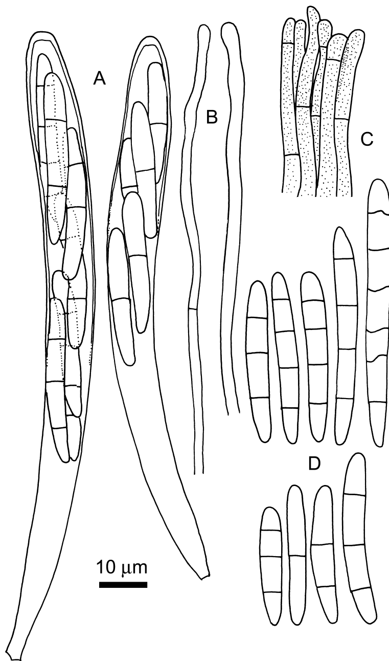
図1. Strossmayeria basitricha . A, 子嚢. B, 側糸. C, 托外被 (縁付近). D, 子嚢胞子.
