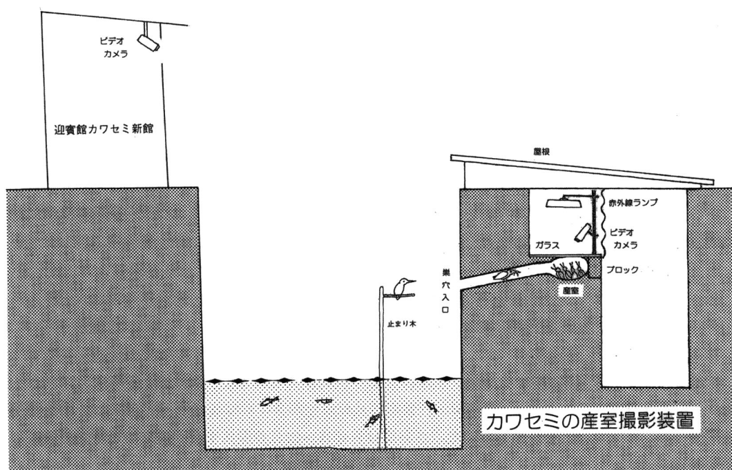
図4. カワセミ繁殖地の撮影機器の配置図
