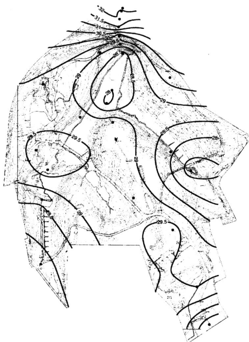
図 3. 2009 年 8 月 16 日 16 時の気温分布
