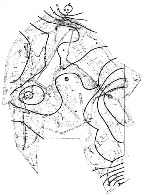
図 2. 2009 年 8 月 16 日 12 時の気温分布
