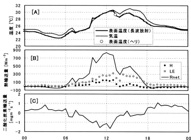
図 9. 樹冠上での[A]温度、[B]熱輸送量、[C]二酸化炭素輸送量、2009 年 8 月 12 日。[A]の丸印はヘリコプターからの測定値。[B]には顕熱輸送量( H )、潜熱輸送量( LE )、正味放射量( R_{net} )を示した。熱輸送量と二酸化炭素輸送量は樹冠から上空へ輸送される場合をプラスとしている。
