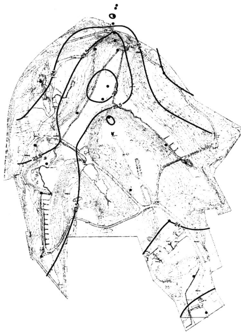
図 5. 2009 年 8 月 17 日 0 時の気温分布
