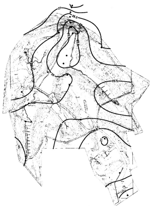
図 4. 2009 年 8 月 16 日 20 時の気温分布
