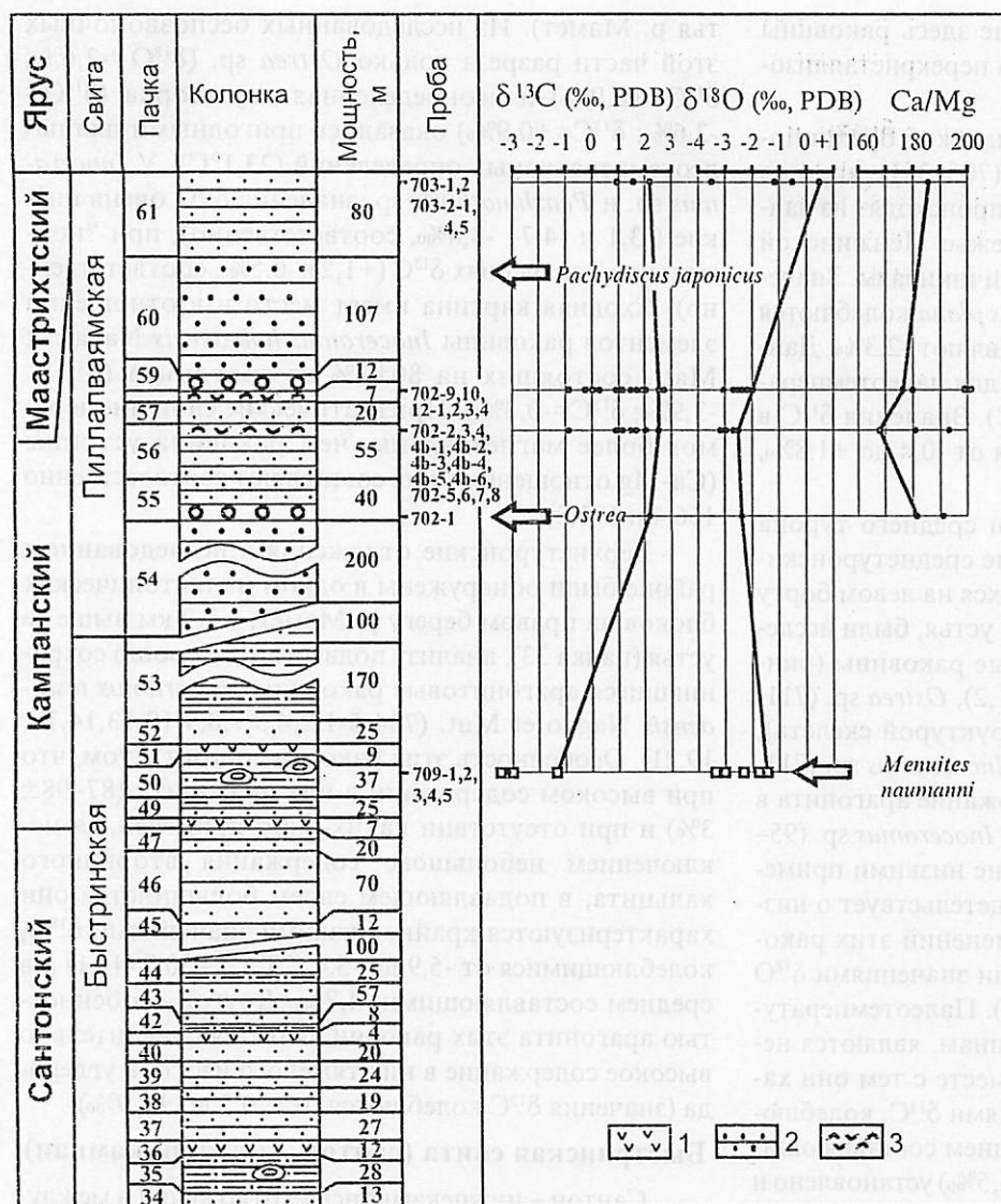
Рис. 5. Соотношения изотопов кислорода и углерода и Ca/Mg отношение в арагонитовых раковинах раннекампанских аммоидей и кальцитовых раковинах позднекампанских двустворок и раннемаастрихтских брахиопод Пенжинской губы.
