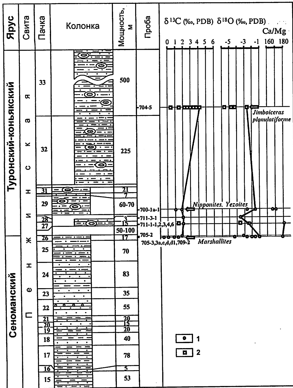
Рис. 4. Соотношения изотопов кислорода и углерода и Ca/Mg отношение в кальцитовом и арагонитовом материале беспозвоночных из верхнего сеномана, турона и сантона Пенжинской губы.
