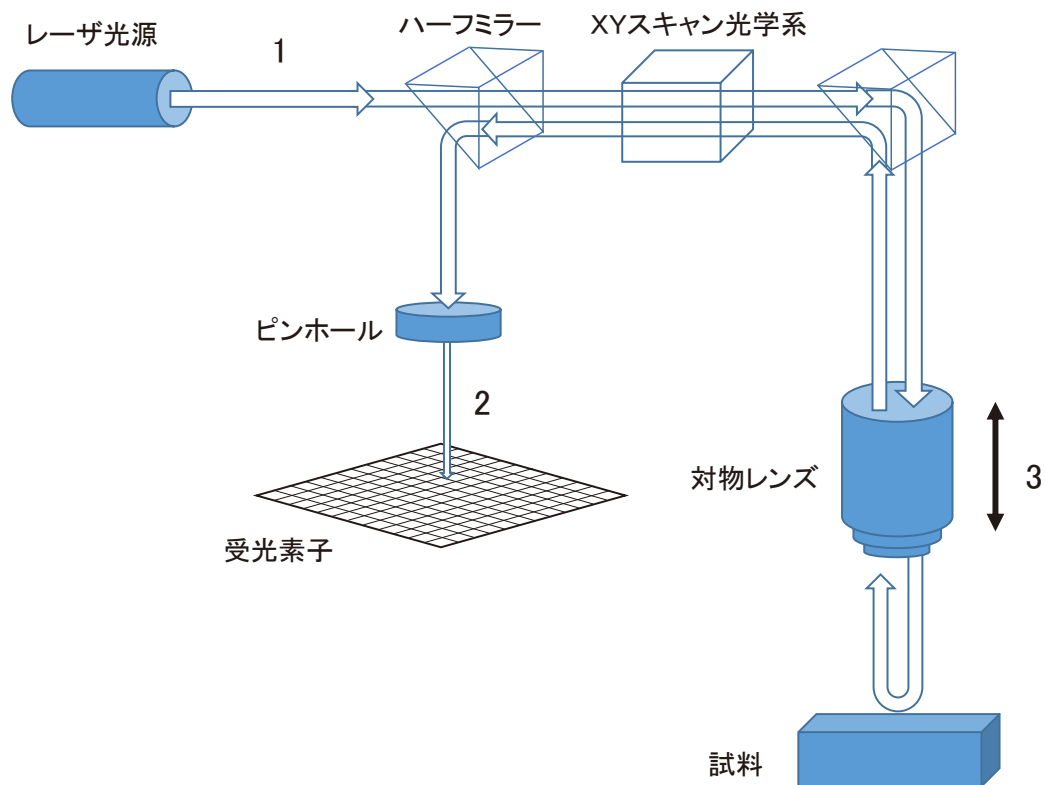
図2. 三次元形状測定装置の測定原理 (キーエンス社資料を基に作成)。1, 光源から照射された光がピクセルに分画された試料表面をXY方向に走査。2, 反射光はピンホールを経由して受光素子に入射し、各ピクセルの反射光量が記録される。3, 全視野をスキャン後、対物レンズの焦点を移動させ、1, 2をZ軸の測定レンジ分繰り返す。4, 各ピクセルについて、反射光量が最大 (=合焦点位置) となるZ軸位置を統合することで、表面の三次元形状を取得。
