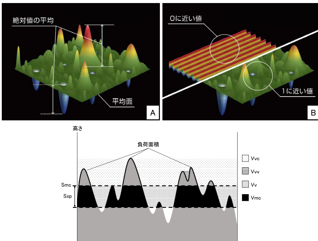
図6. ISO パラメータが抽出する形態学的特徴の模式図（キーエンス社資料を改変）。A, Sa（各測定点の平均面に対する距離の平均）。B, Str（形状の規則性・筋目の有無）。C, 機能パラメータ（Smc, Sxp）および体積パラメータ（Vmc, Vvc, Vv, Vvv）。定義は本文を参照。便宜上，立体断面を示す。なお，実際のSmcとSxpの算出に用いる高さは異なる。
