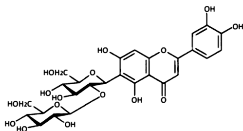
Fig. 10. Isoorientin 2''-O-glucoside ( CF9 ).
