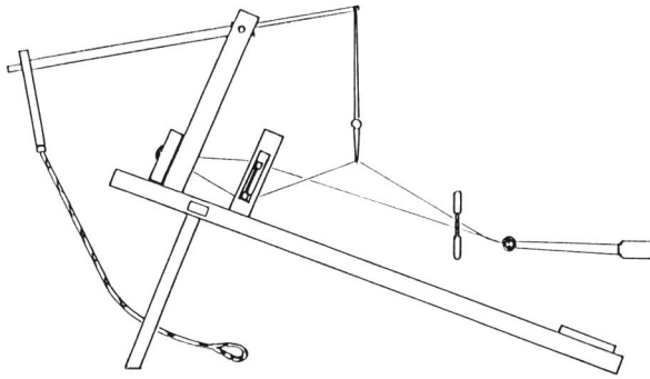
傾斜型地機
