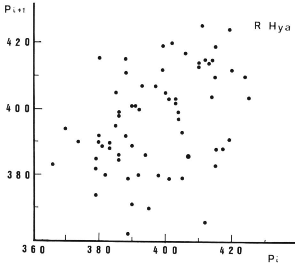
Fig. 4. First return map of R Hya.
