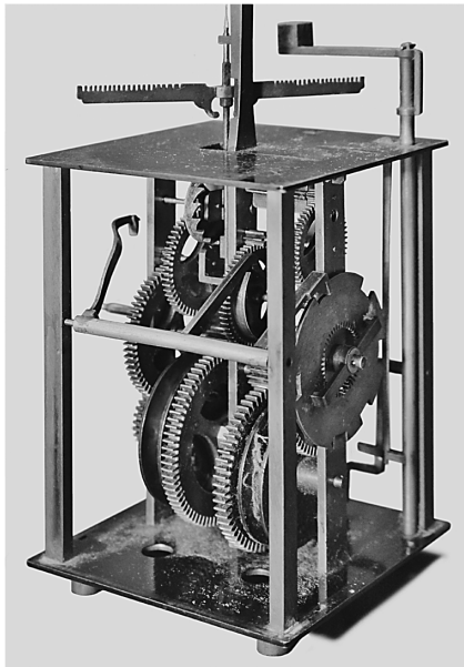
写真8. 時計機構（右後方から）
