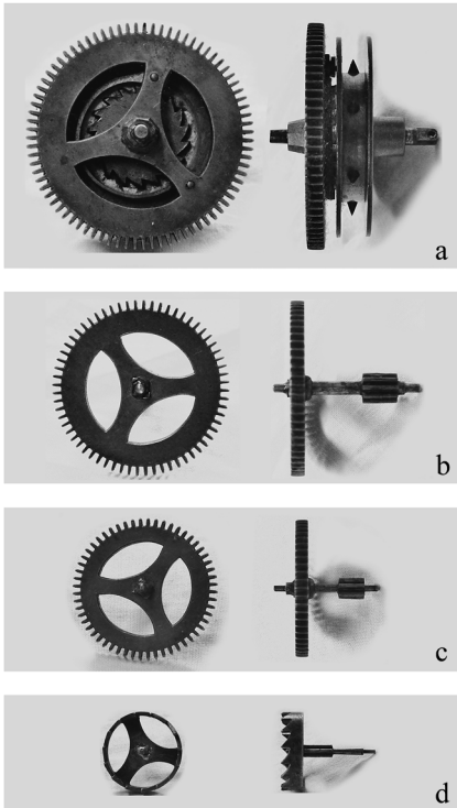
写真10. 時方輪列
