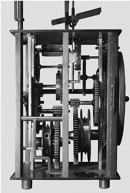
写真7. 時計機構（左側面）
