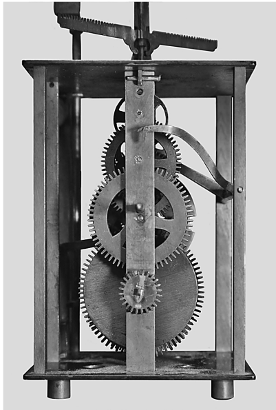
写真4. 時計機構（正面）
