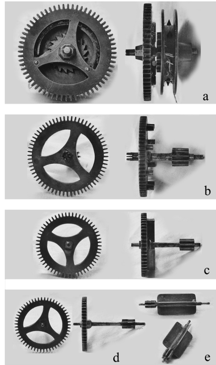
写真11. 打方輪列
