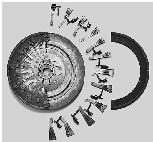
写真18. 分解した文字盤
