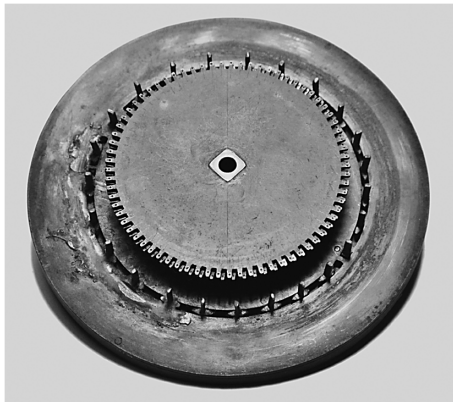
写真15. 文字盤（裏面）
