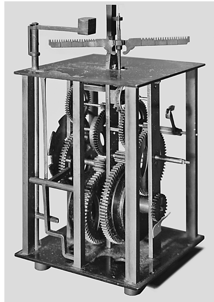
写真9. 時計機構（左前方から）
