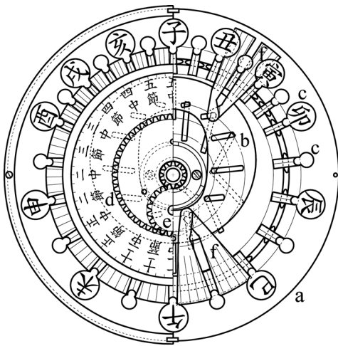
図2. 在政の自動割駒式文字盤
