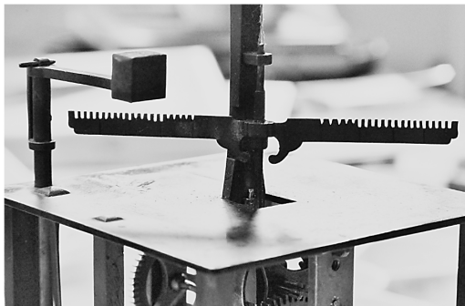
写真12. 一挺天符
