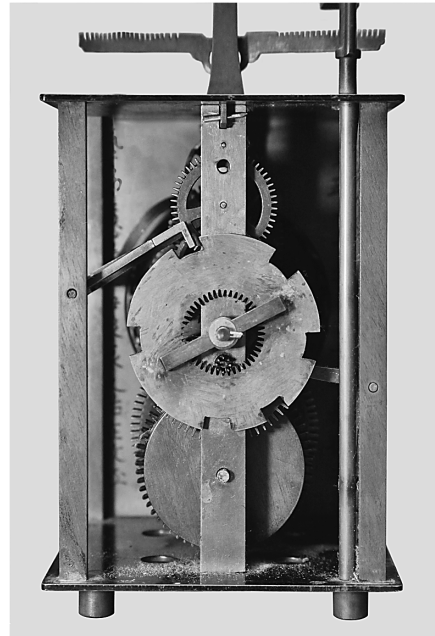
写真6. 時計機構（背面）
