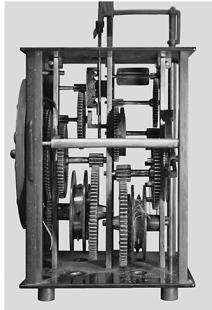
写真5. 時計機構（右側面）
