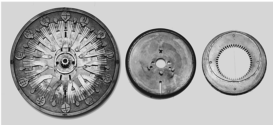
写真17. 文字盤，節気目盛盤ケース，年周カム（節気目盛盤）
