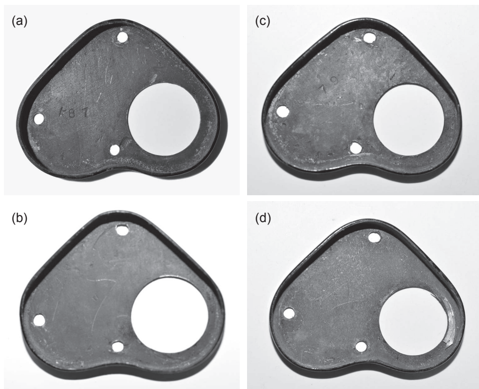
図5 接眼側鏡体カバー内面部 (a)寄贈機, (b)N氏所蔵機, (c)中島2号機, (d)同1号機
