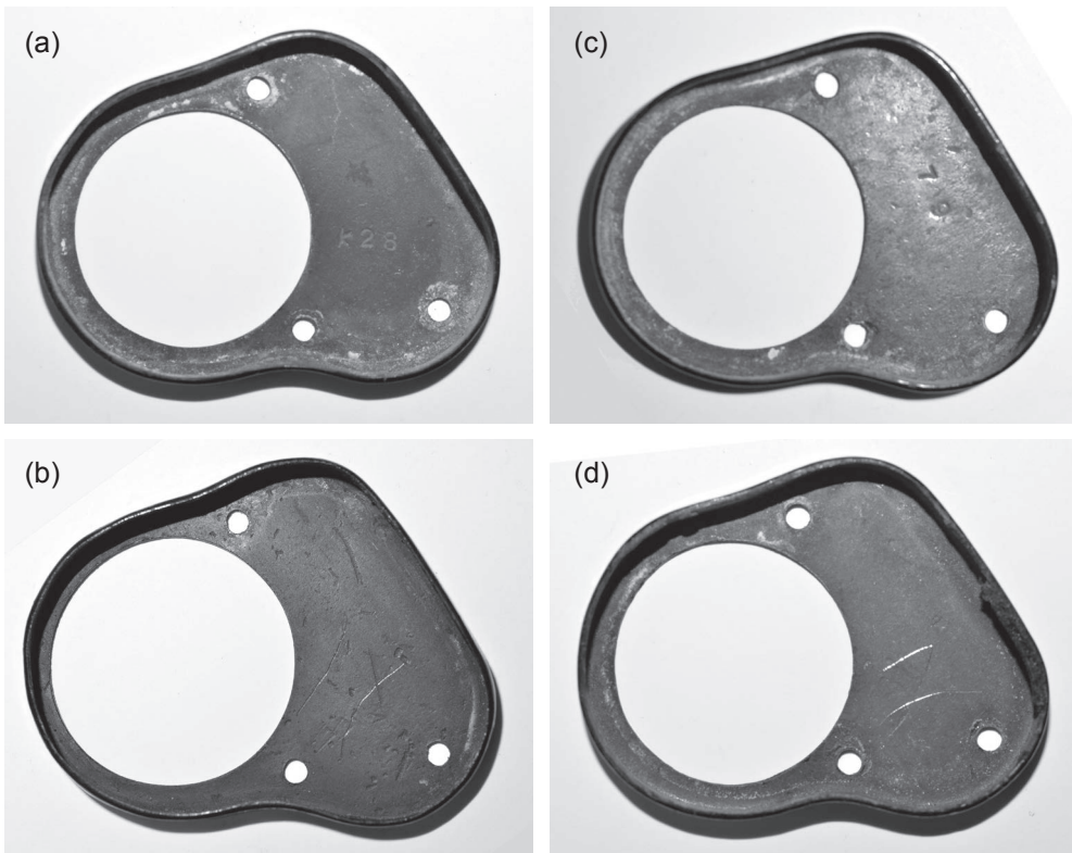
図4 対物側鏡体カバー内面部 (a)寄贈機, (b)N氏所蔵機, (c)中島2号機, (d)同1号機
