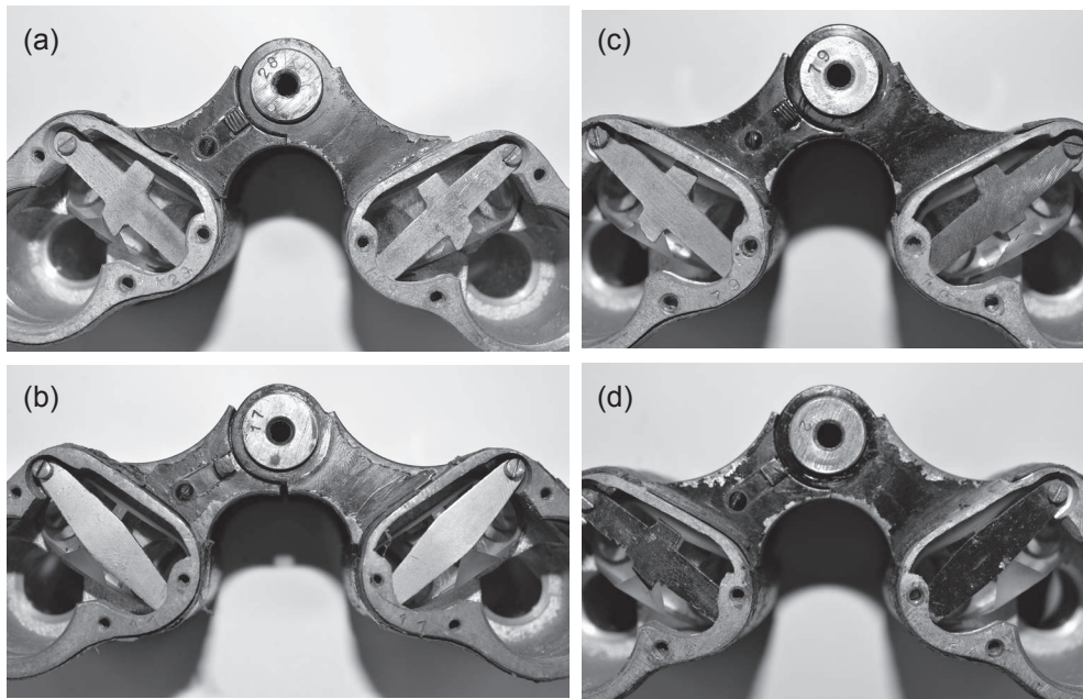
図3 中心軸金具と鏡体対物側の端面部 (a)寄贈機, (b)N氏所蔵機, (c)中島2号機, (d)同1号機
