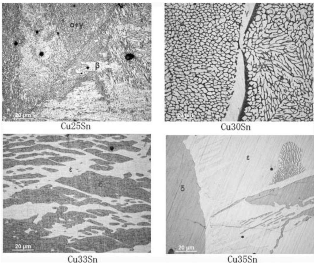
図8. Cu25Sn, Cu30Sn, Cu33Sn (国友鏡相当), Cu35Sn合金のSEMによる725倍金属組織写真。
