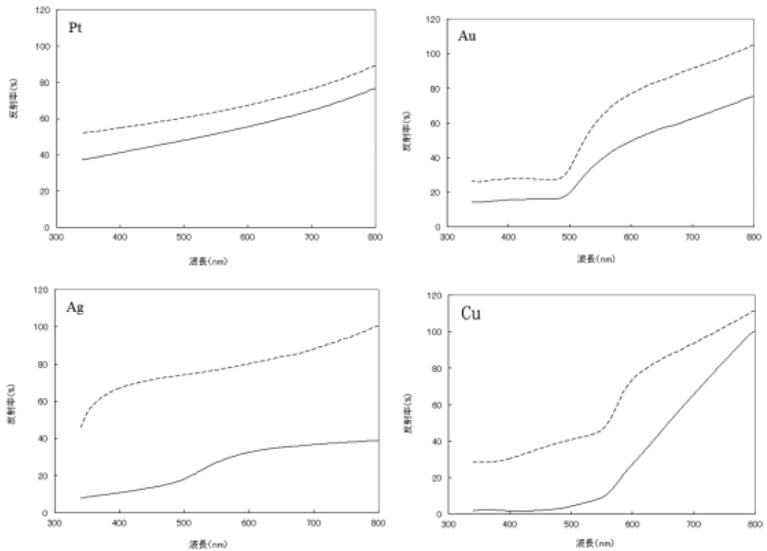
図3. 純金属Pt, Au, Ag, Cuの分光反射率. 実線は10年経過後の表面, 破線は新しい研磨面を示す.
