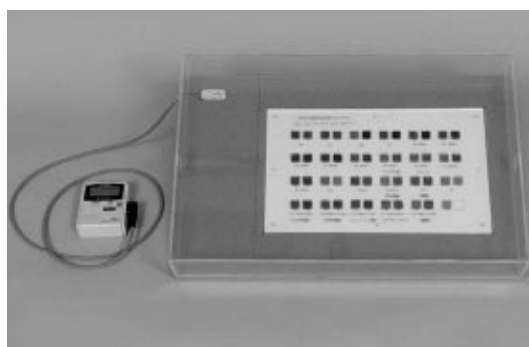
図2. 23種の金属試料を並べた耐環境試験用の収納ケースと温湿度データロガー. 右下隅には分光測定用比較試料のAl真空蒸着ガラス鏡が1片置いてある.
