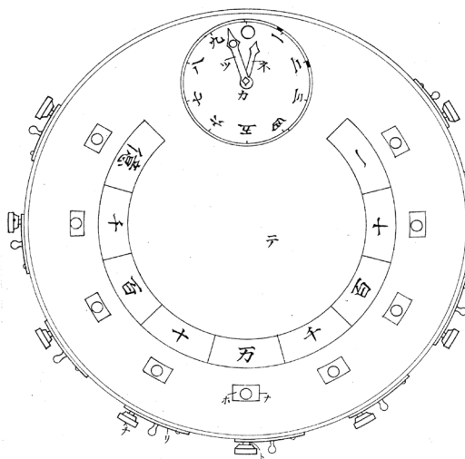
(b)正面図
