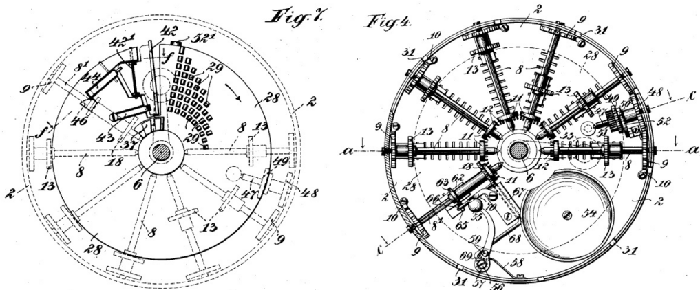
(a) 平面図
