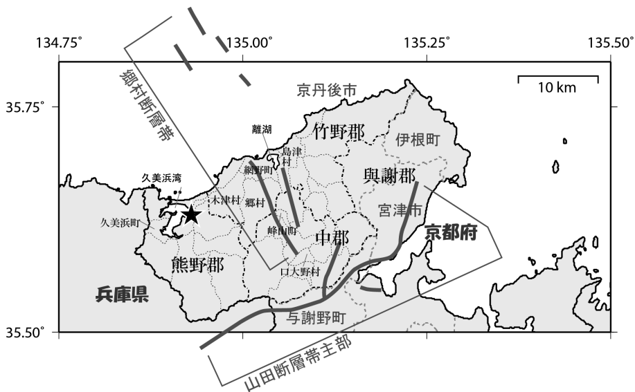
図1. 山田断層帯と京都府北部の行政区。山田断層帯を表す灰色太線は地震調査研究推進本部の長期評価 2) による。黒線は県境界、一点鎖線と灰点線はそれぞれ1927年の郡境界と町村境界、灰破線は現在の市町郡境界を表し、ゴシック体で地名を示した。明朝体は1927年の地名。今回の写真に関係ある町村のみ示す。黒星は気象庁による1927年北丹後地震の震央を示す。
