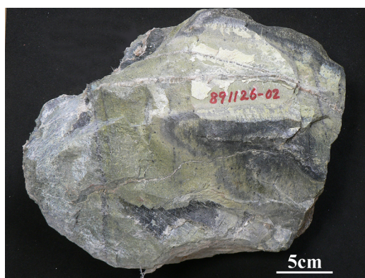
Fig. 10. Serpentinite from Mineração de Amianto at Mina da Cana Brava, Minaçu (GO).
