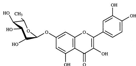
Fig. 3. Quercetin 7- O -rhamnoside (Vincetoxicoside B, 4 ).
