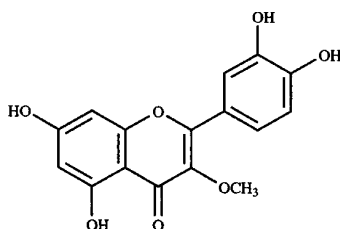
Fig. 6. Quercetin 3-methyl ether ( 7 ).
