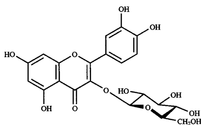
Fig. 2. Quercetin 3- O -glucoside (Isoquercitrin, 3 ).
