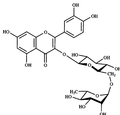
Fig. 4. Quercetin 3- O -rutinoside (Rutin, 5 ).
