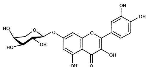
Fig. 1. Quercetin 7- O -arabinoside ( 2 ).
