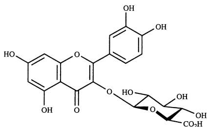
Fig. 5. Quercetin 3- O -glucuronide (Miquelianin, 6 ).
