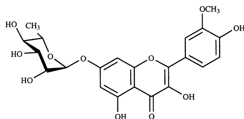
Fig. 9. Isorhamnetin 7- O -rhamnoside ( 10 ).
