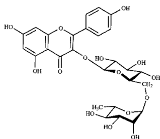
Fig. 10. Kaempferol 3- O -rutinoside ( F5 ).
