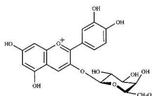
Fig. 3. Cyanidin 3- O -galactoside ( A3 ).
