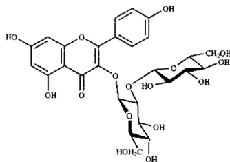
Fig. 8. Kaempferol 3- O -sophoroside ( F3 ).
