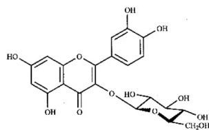
Fig. 6. Quercetin 3- O -glucoside ( F1 ).
