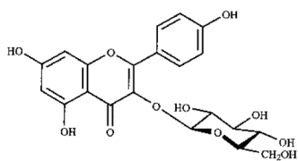
Fig. 9. Kaempferol 3- O -glucoside ( F4 ).
