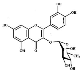
Fig. 11. Quercetin 3- O -rhamnoside ( F6 ).
