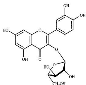
Fig. 12. Quercetin 3- O -arabinofuranoside ( F7 ).
