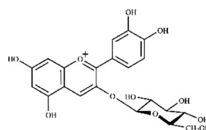
Fig. 4. Cyanidin 3- O -glucoside ( A4 ).
