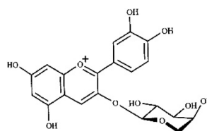
Fig. 5. Cyanidin 3- O -arabinoside ( A5 ).
