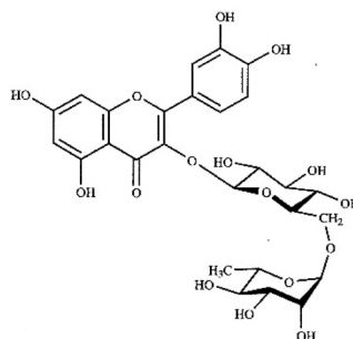
Fig. 7. Quercetin 3- O -rutinoside ( F2 ).
