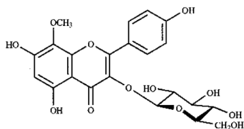
Fig. 13. Sexangularetin 3- O -glucoside ( F8 ).
