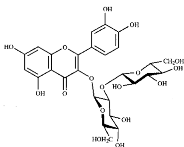
Fig. 14. Quercetin 3- O -sophoroside ( F9 ).
