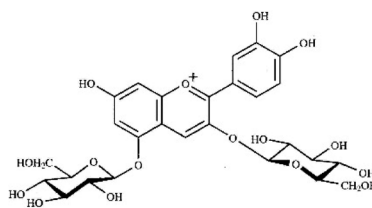
Fig. 2. Cyanidin 3,5-di- O -glucoside ( A2 ).
