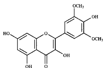
Fig. 10. Syringetin.
