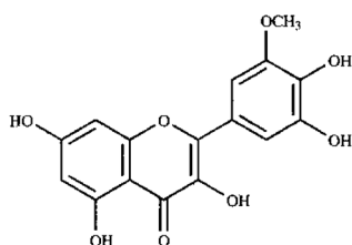
Fig. 9. Laricitrin.
